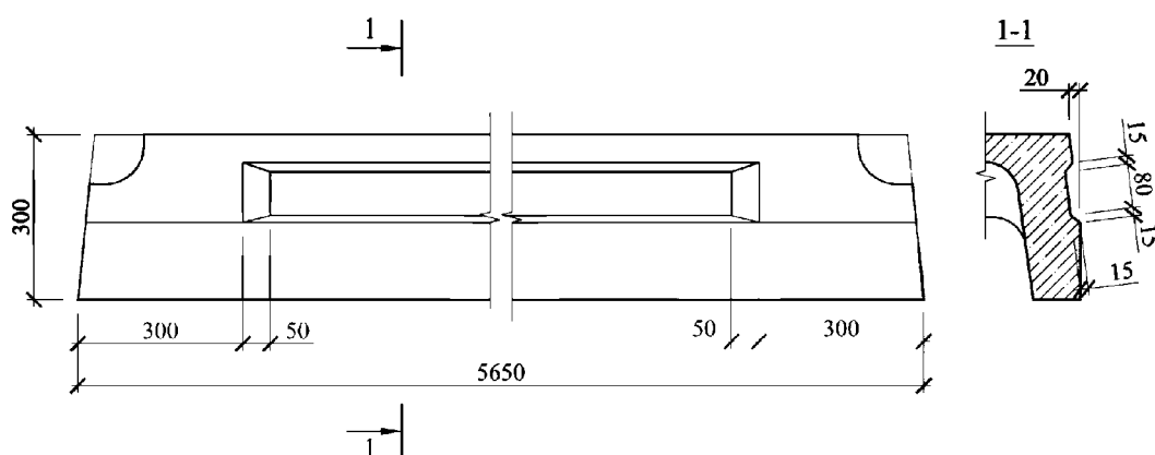
Рисунок 1. Углубление на боковой поверхности плиты
